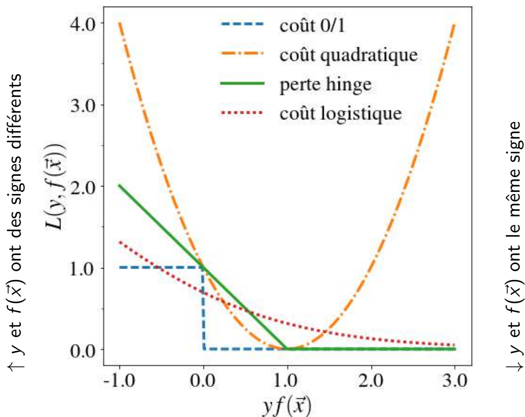
FIGURE 2.4 – Fonctions de perte pour la classification binaire.
