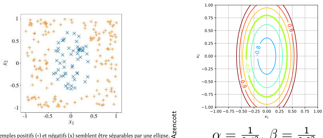
FIGURE 2.2 – Les exemples positifs (+) et négatifs (x) semblent être séparables par une ellipse.
