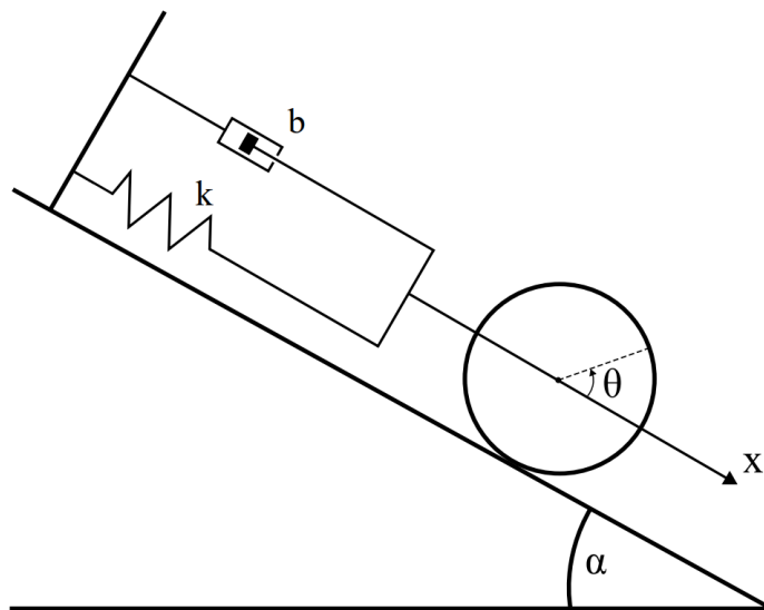
FIGURE 1 – Cylindre de masse M sur un plan incliné d'angle \alpha par rapport à l'horizontal, maintenu en son centre de masse G par un ressort ainsi qu'un amortisseur tous deux reliés à une paroi rigide.
