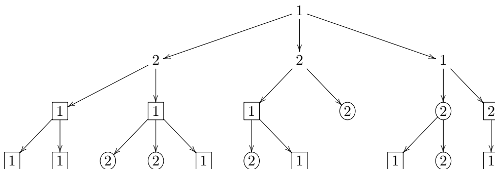
FIG. 3: Lorsque g est définie sur les nœuds de hauteur > k , nous pouvons la définir sur les nœuds de hauteur k .
