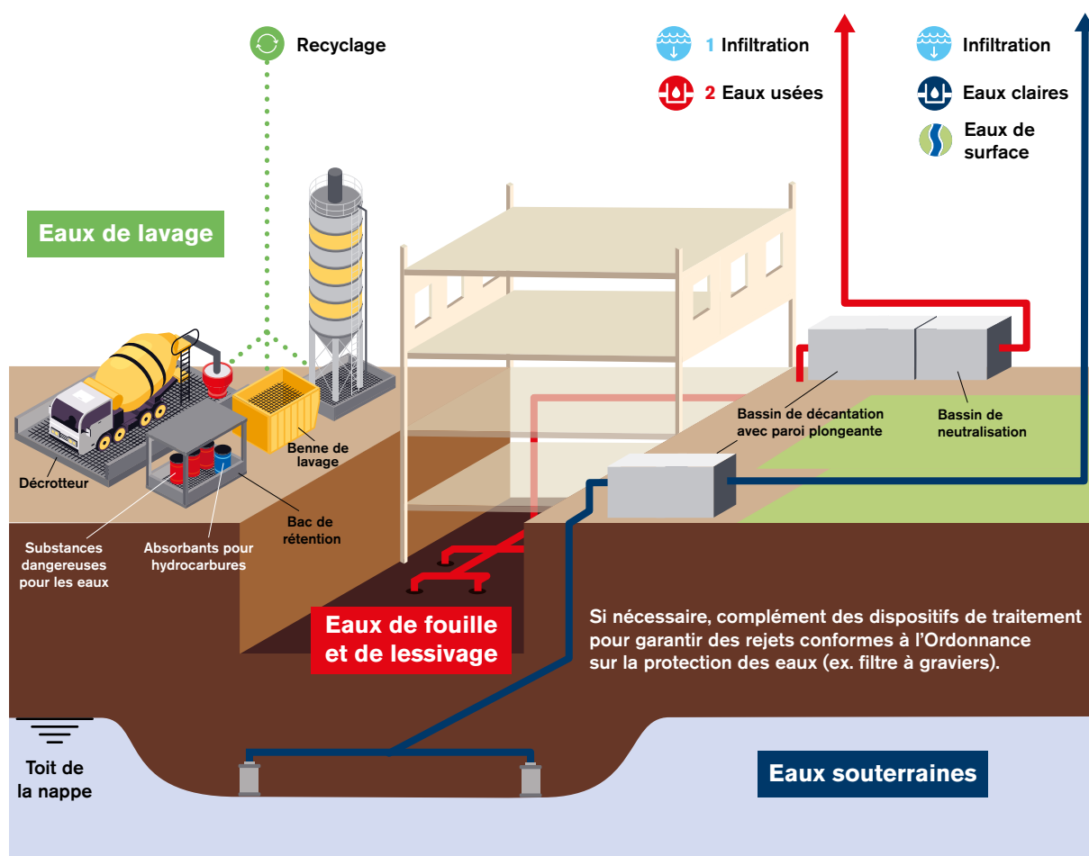
Schéma 2 : Illustration des principes de la gestion des eaux de chantier pour les projets de la construction.
