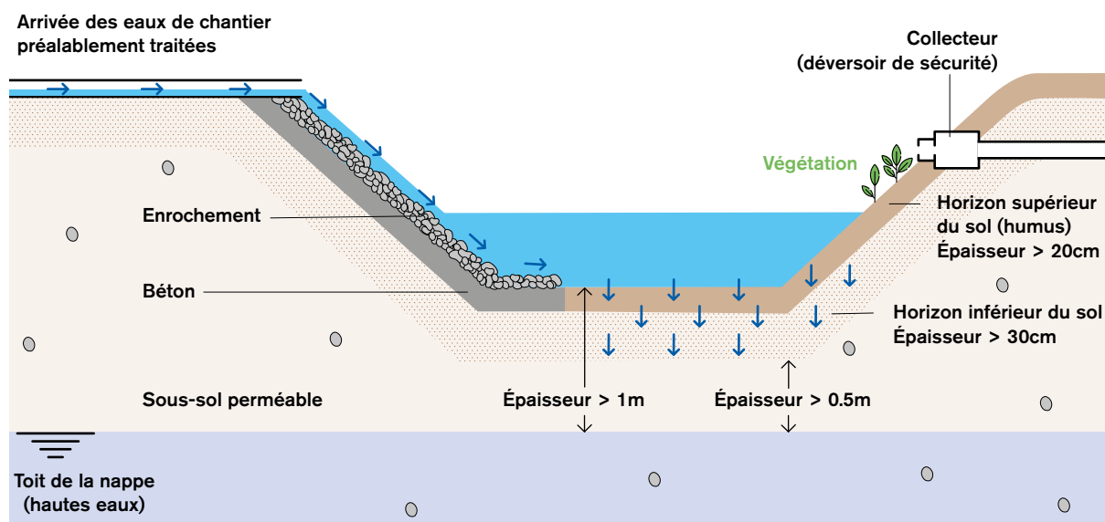
Schéma 3 : Illustration du principe d'infiltration.
