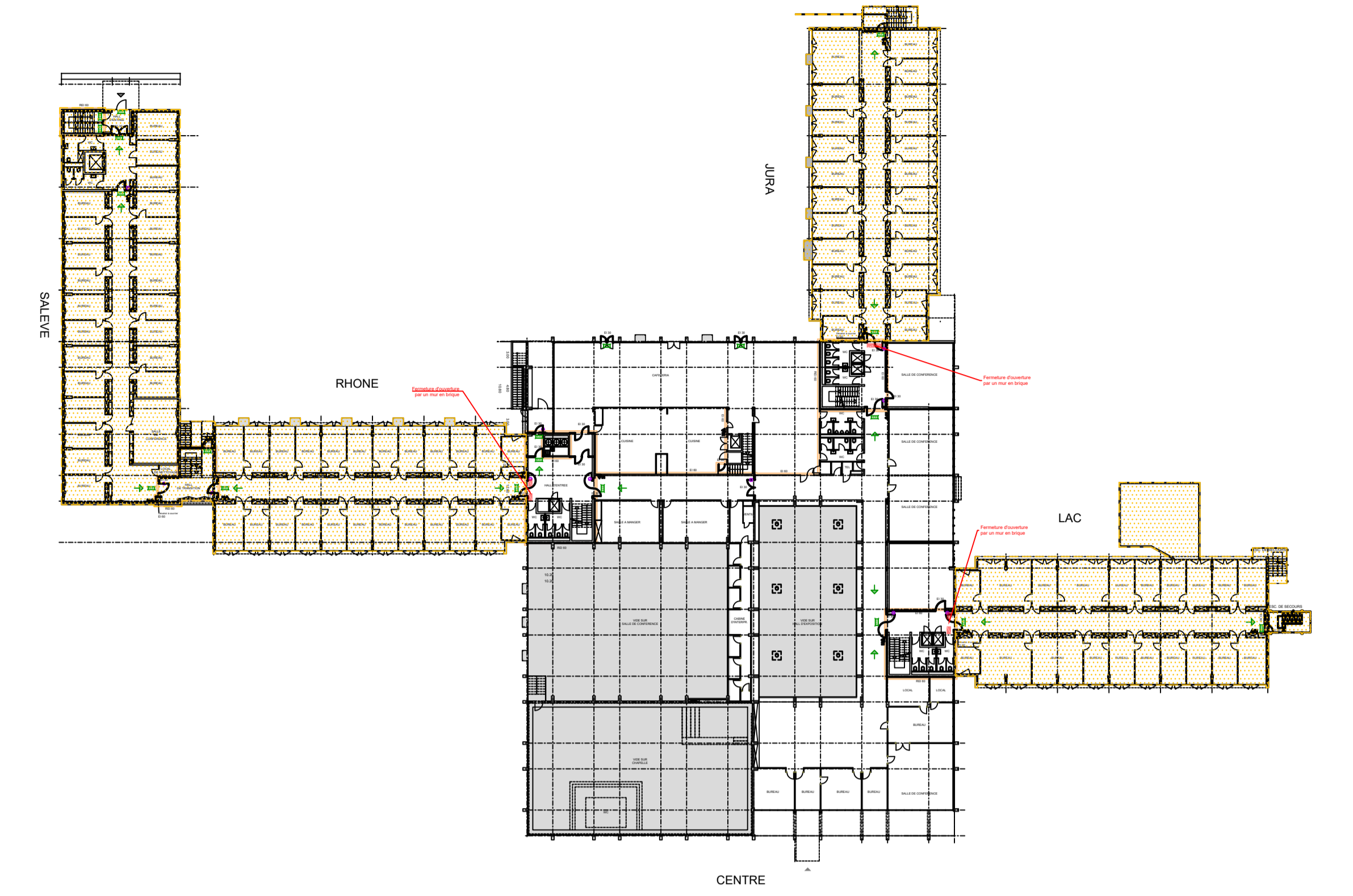
Vue en plan Rez-supérieur Ech: 1/500
