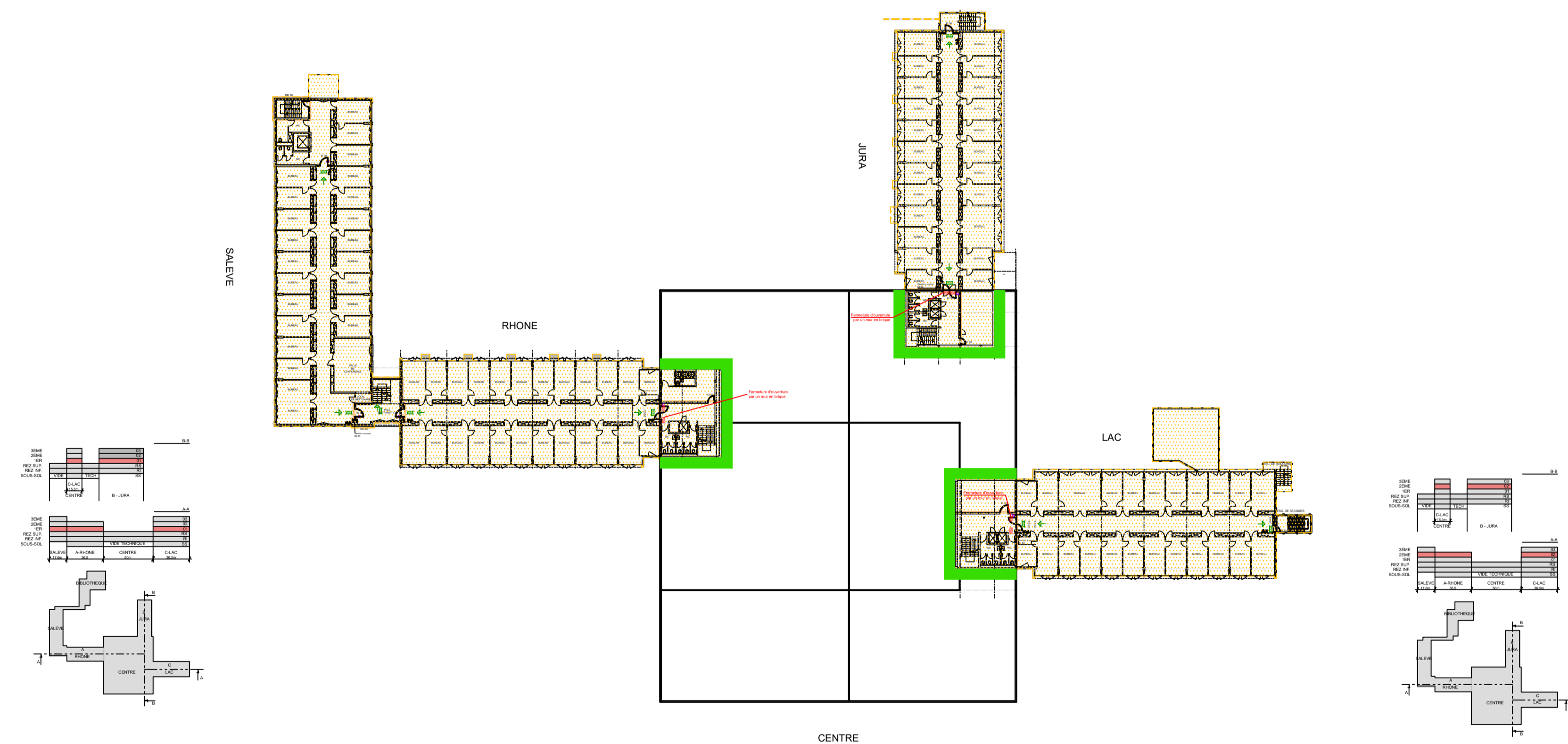
Vue en plan 1ère étage Ech: 1/500
