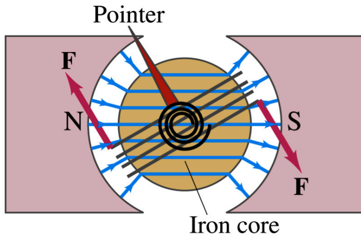
Galvanometer
