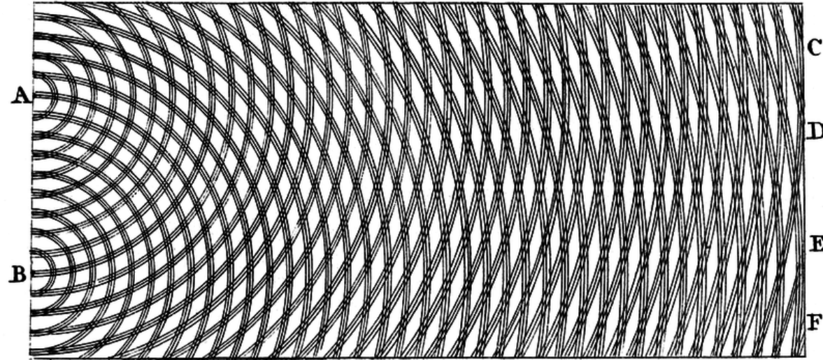
Dessin original de Thomas Yung pour la diffraction par deux fentes
