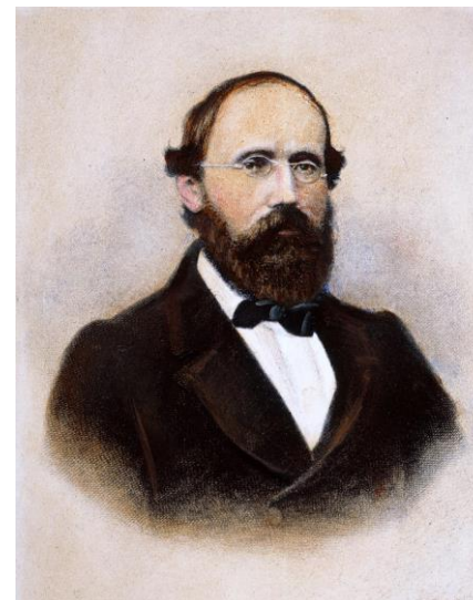
Bernhard Riemann
