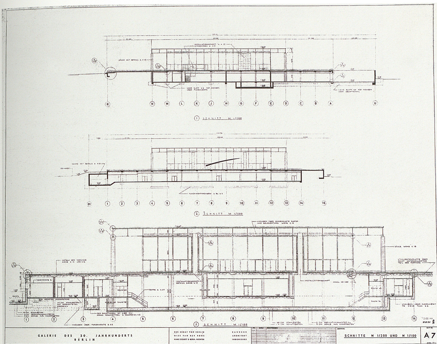
Abb. 77 Neue Nationalgalerie Berlin, 3 Schnitte
