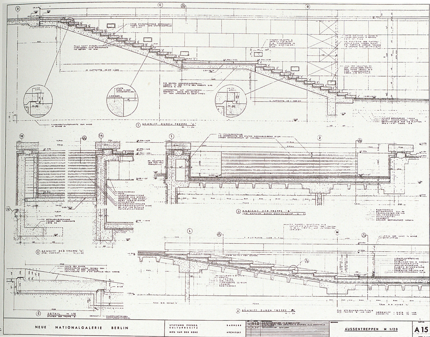
Abb. 79 Neue Nationalgalerie Berlin, Detail der Außentreppe
