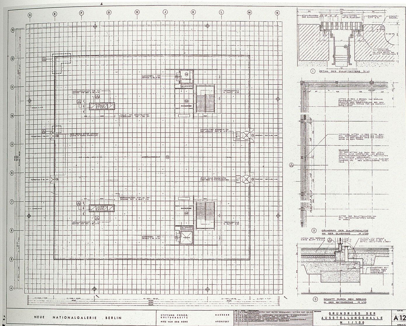
Abb. 76 Neue Nationalgalerie Berlin, Grundriß der Ausstellungshalle mit Details
