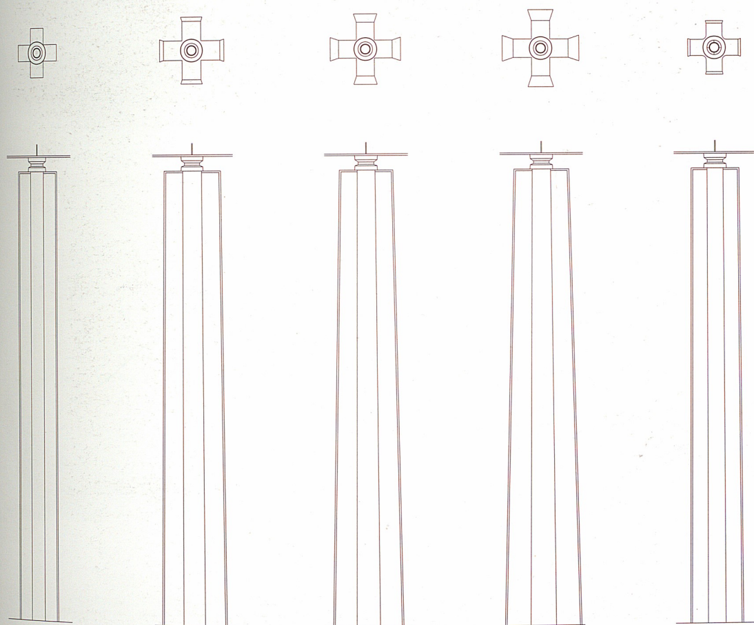
Abb. 75 Neue Nationalgalerie Berlin, Modellvarianten der Stahlstützen. Die Variante rechts kam zur Ausführung.
