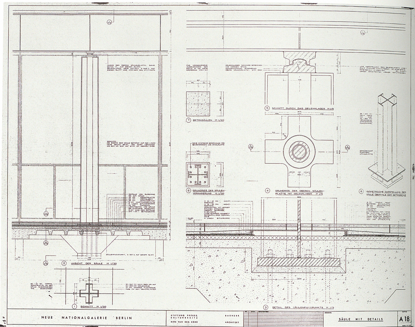
Abb. 78 Neue Nationalgalerie Berlin, Stütze und Details
